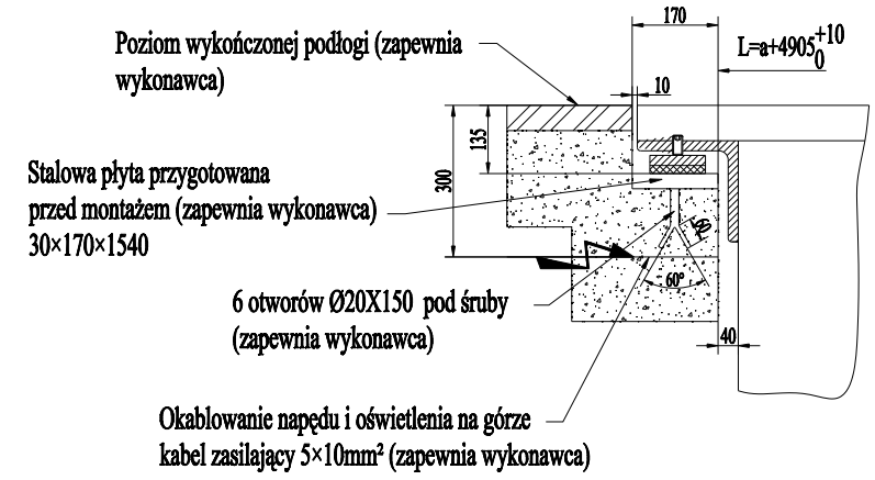
Szczegół A
